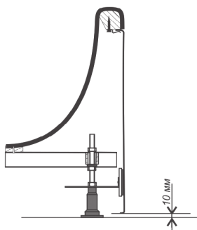
Рис. 1. Установка ванны по высоте.
