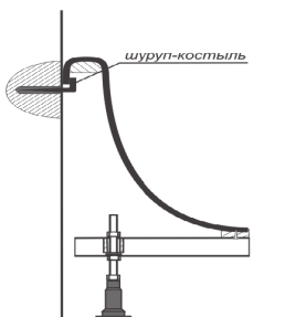
Рис. 2. Установка ванны на скобы.
