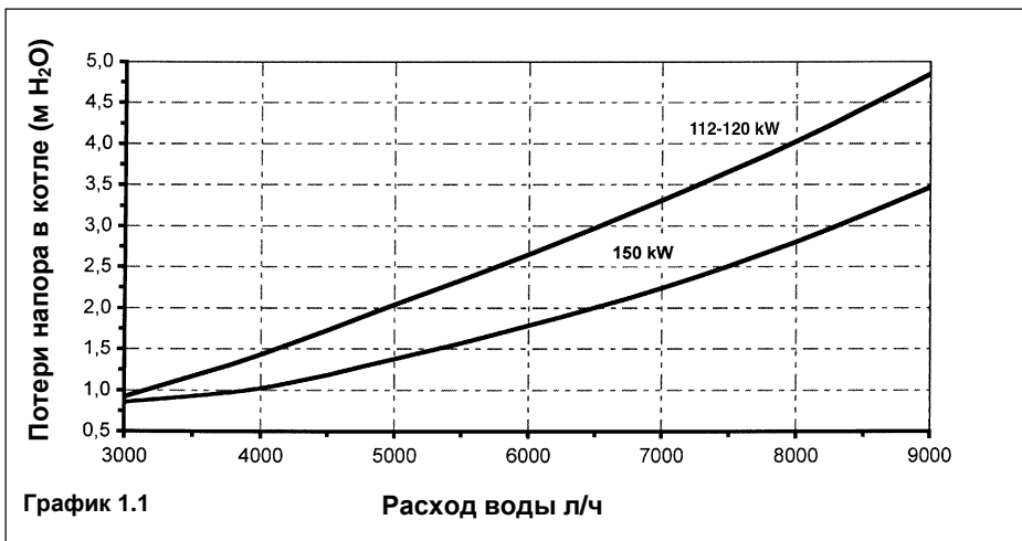
ПОТЕРИ НАПОРА В КОТЛАХ МОДЕЛЕЙ POWER HT 1.1200 – 1.1500
