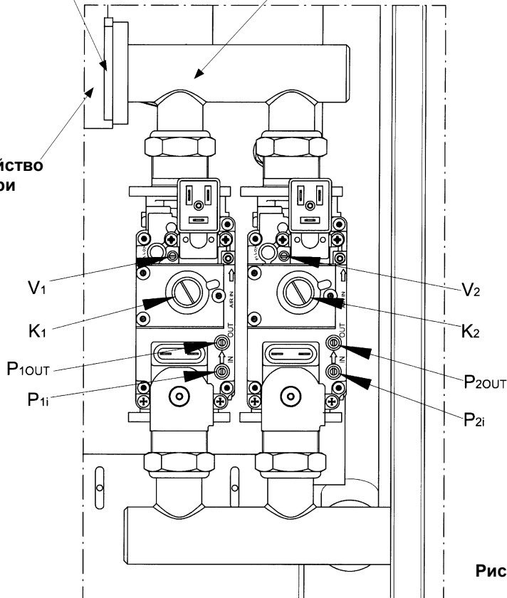
Газовая диафрагма
